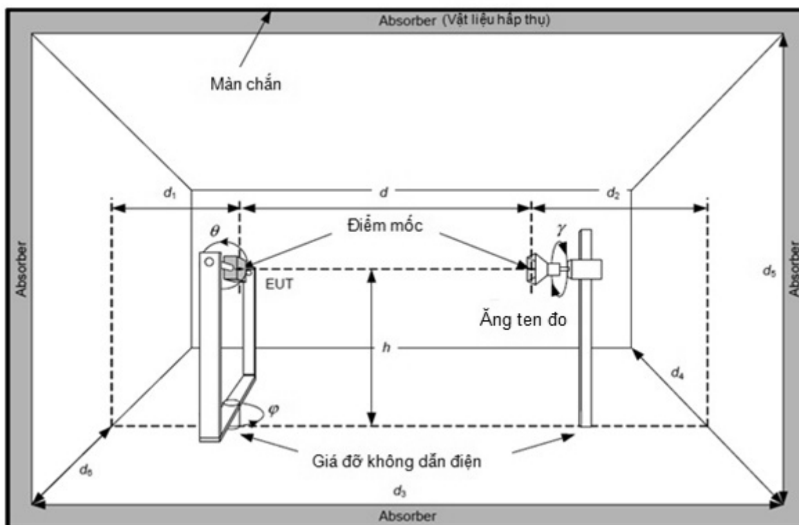
Hình B.5 - Phòng đo kiểm triệt phản xạ điển hình
