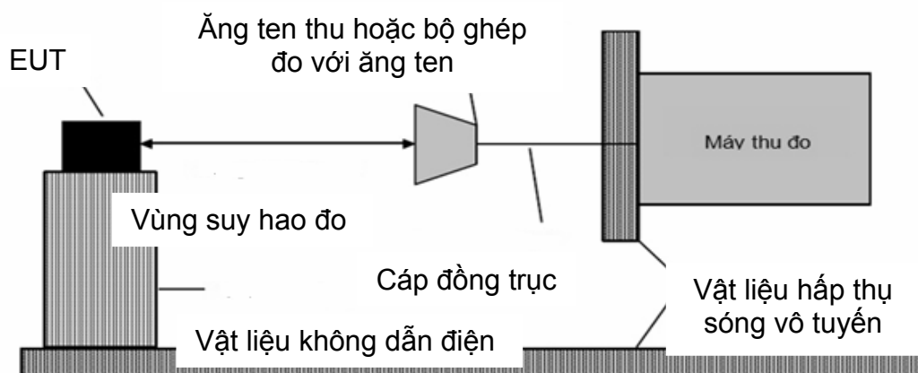
Hình B.6 - Ví dụ về vị trí đo trên 18 GHz với một bề mặt phản xạ
