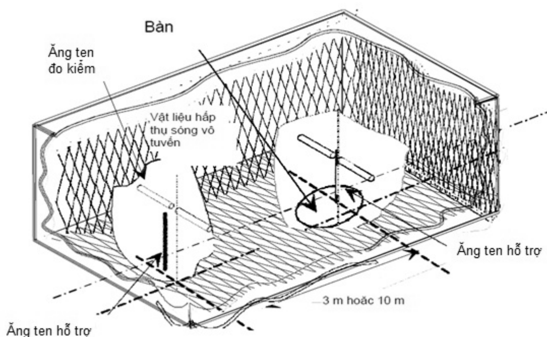
Hình B.4 - Phòng đo kiểm triệt phản xạ điện hình
