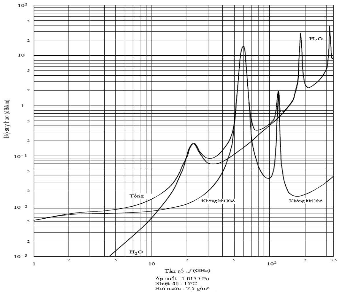
Hình C.1 - Độ suy hao qua không khí trong băng tần 1 GHz đến 350 GHz (dB/km)
