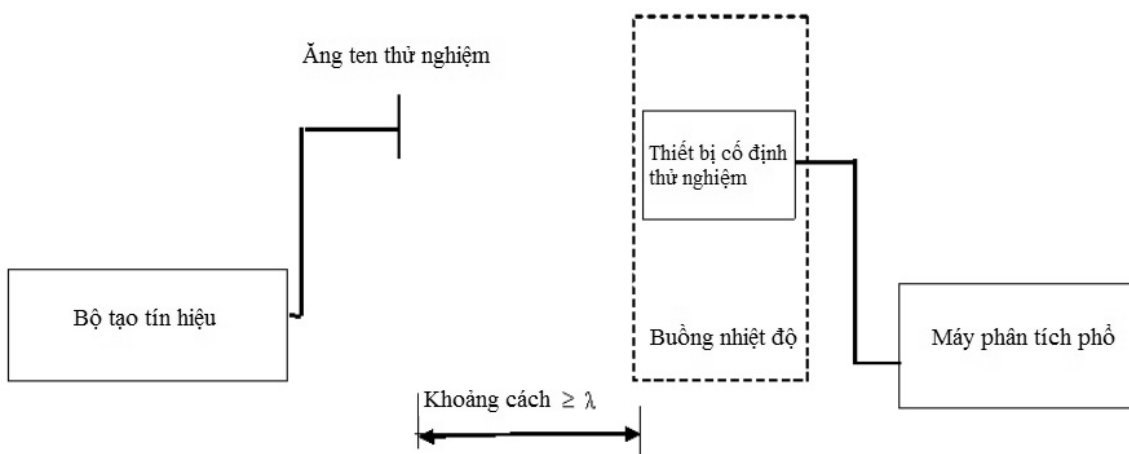
Hình C.5 - Xác nhận thiết bị cố định thử nghiệm không cần EUT
