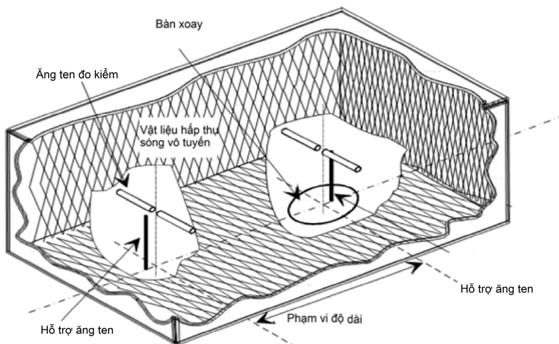
Hình C.1 - Phòng đo kiểm không phản xạ điển hình
