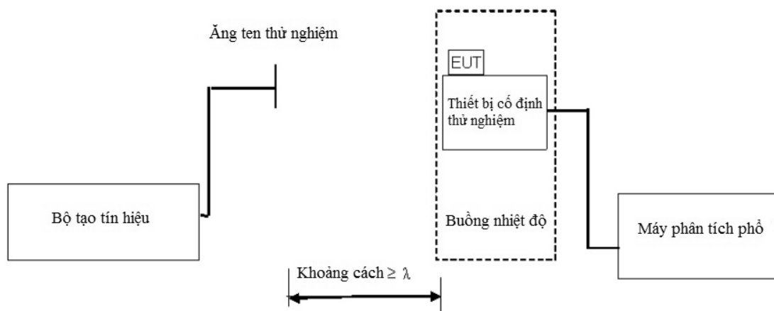
Hình C.6 - Xác nhận thiết bị cố định thử nghiệm với EUT đặt tại chỗ
