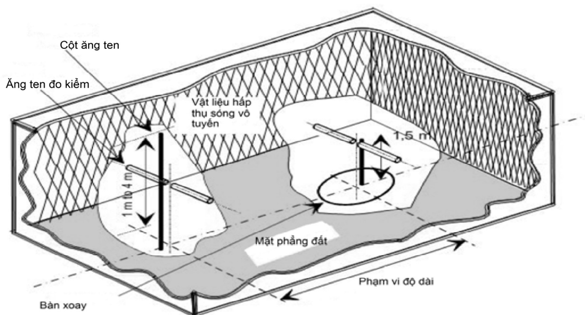
Hình C.2 - Phòng đo kiểm không phản xạ với mặt phẳng dẫn điện hình
