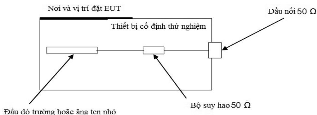
Hình C.4 - Thiết bị cố định thử nghiệm
