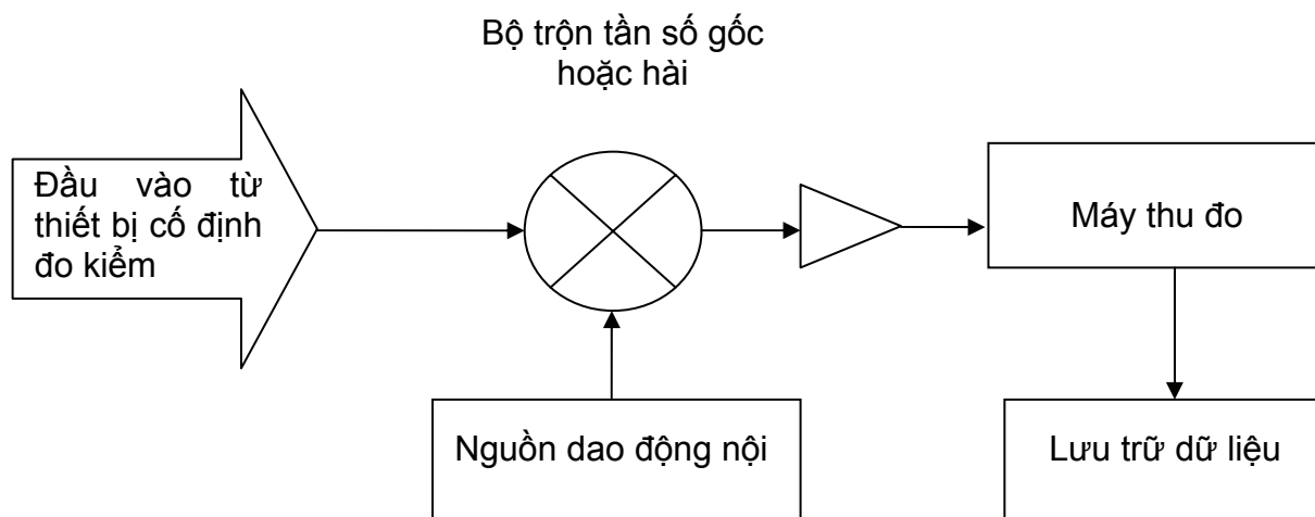
Hình 2 - Sơ đồ thiết lập đo kiểm của bức xạ ngoài băng và phát xạ giả
