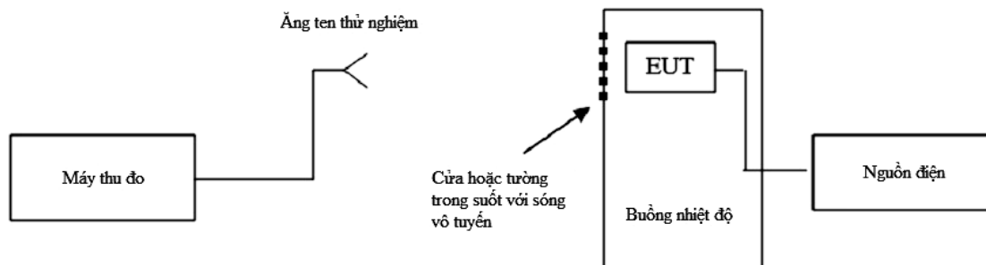
Hình C.3 - Thiết lập điều kiện đo kiểm khắc nghiệt
