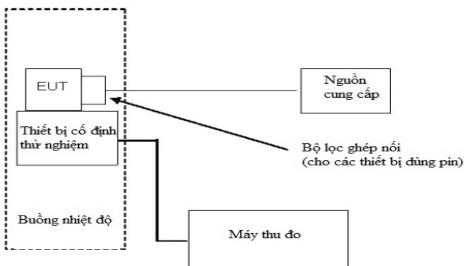
Hình C.7 - Đo EUT thực hiện trong buồng nhiệt độ
