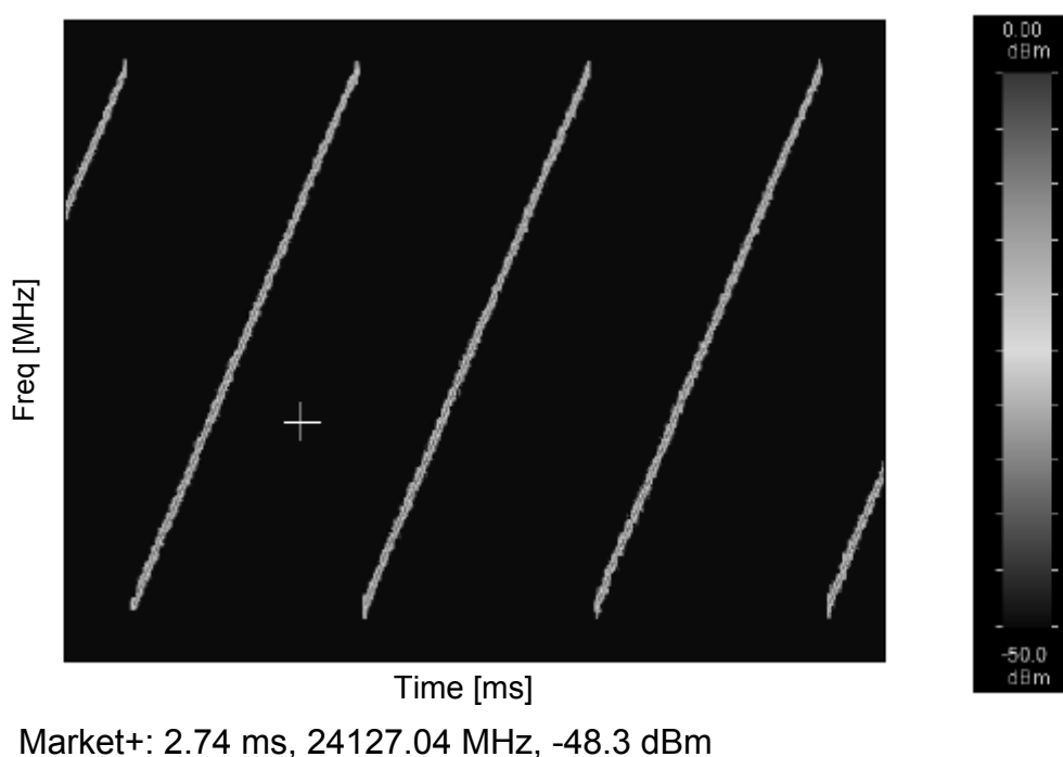
Hình F.2 - Ví dụ về kết quả đo bằng biểu đồ phổ
