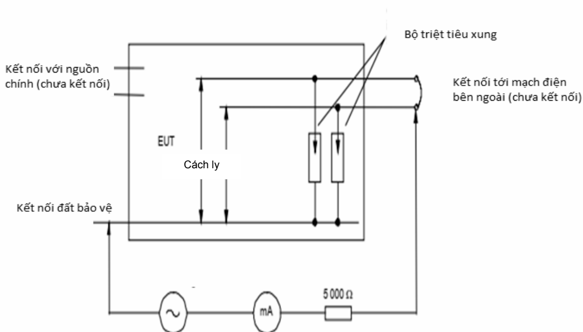
[Hình 31] - Thử nghiệm sự cách ly giữa mạch ngoài và đất
