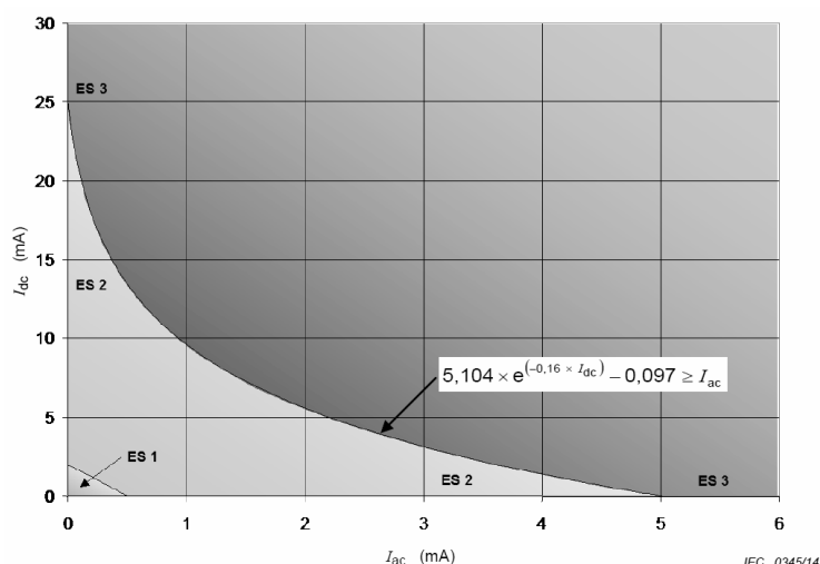
[Hình 22] - Các giá trị cực đại cho kết hợp dòng a.c. và dòng d.c
